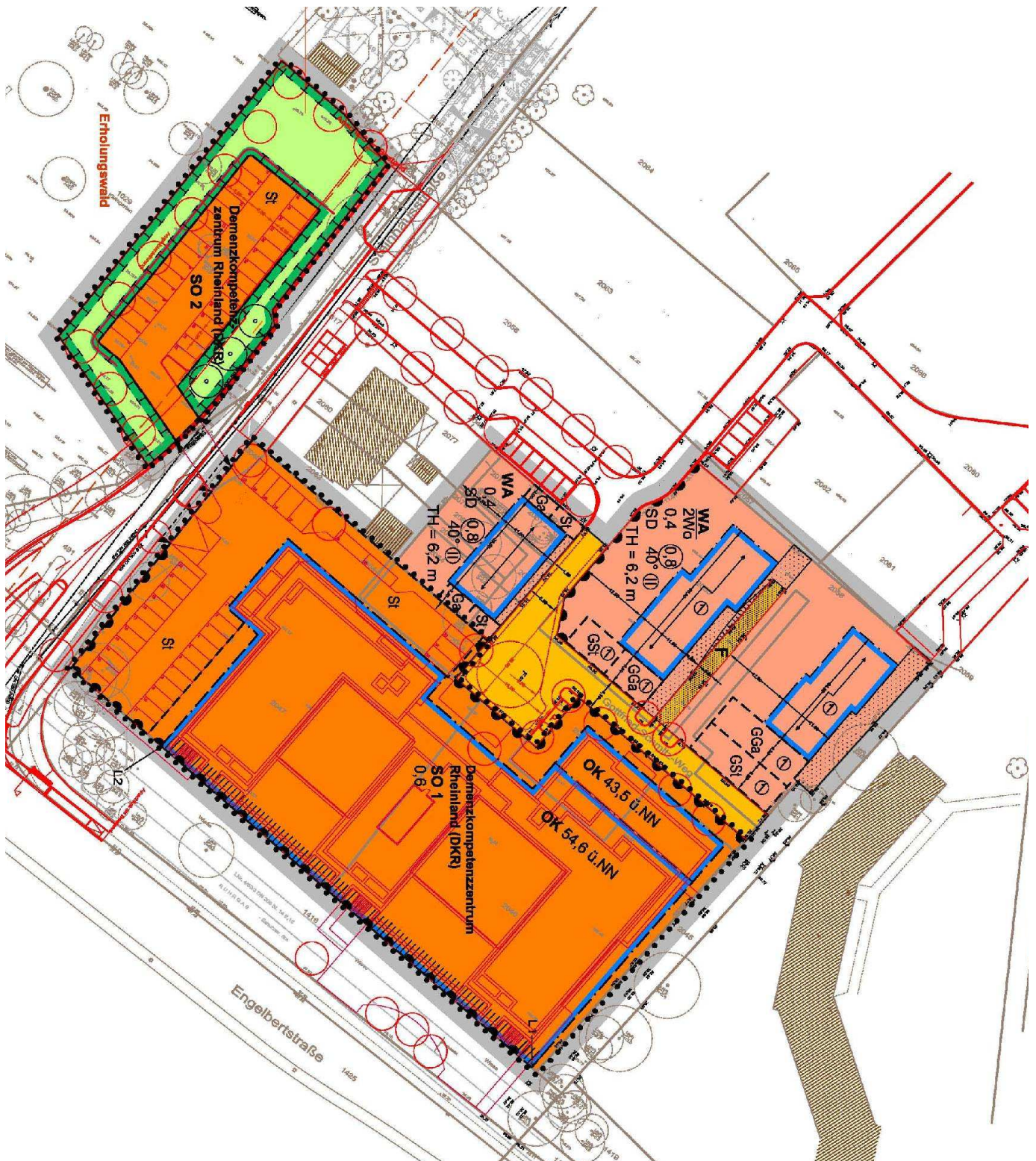
Abb. Verkleinerung der Planzeichnung des Vorhabenbezogenen Bebauungsplans Nr. V 43/11 – Furth-Mitte, Engelbertstraße (Demenzkompetenzzentrum Rheinland) – ohne Maßstab
